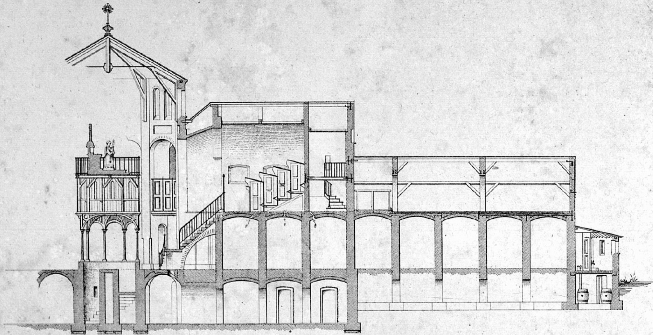
Coupe longitudinale d'une aile et chapelle.
