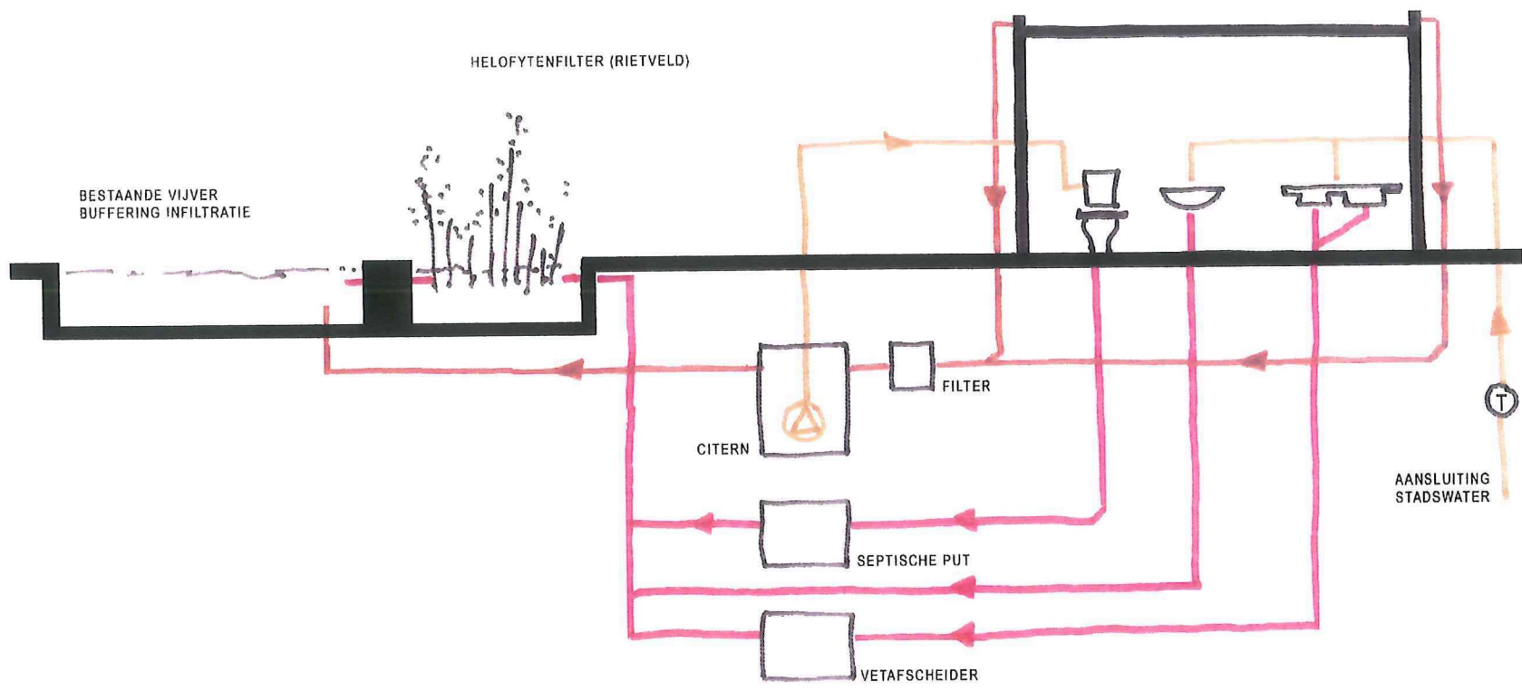
voorstel afvalwaterzuivering
