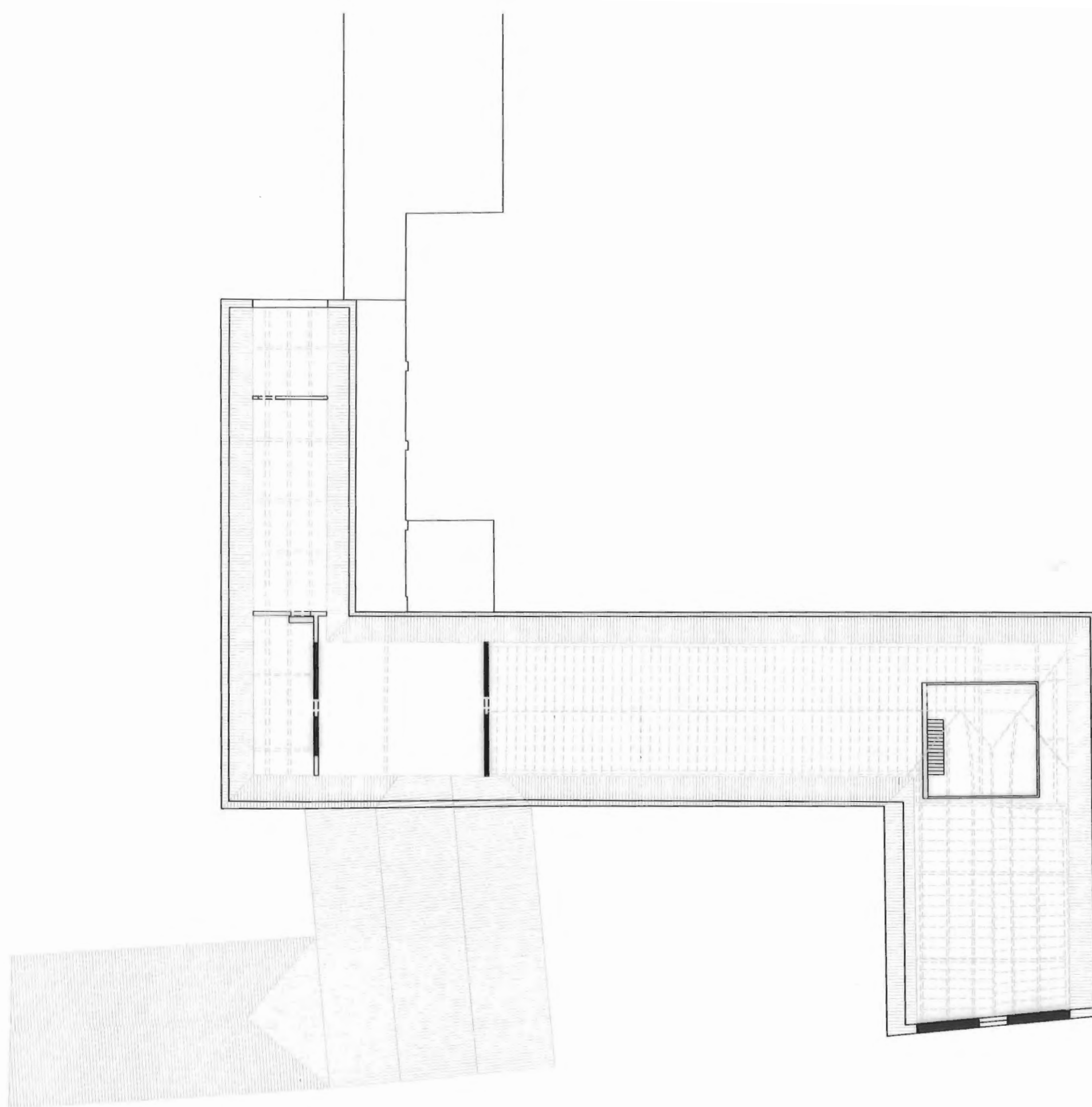
PLAN NIVEAU 2 - te behouden structuur
