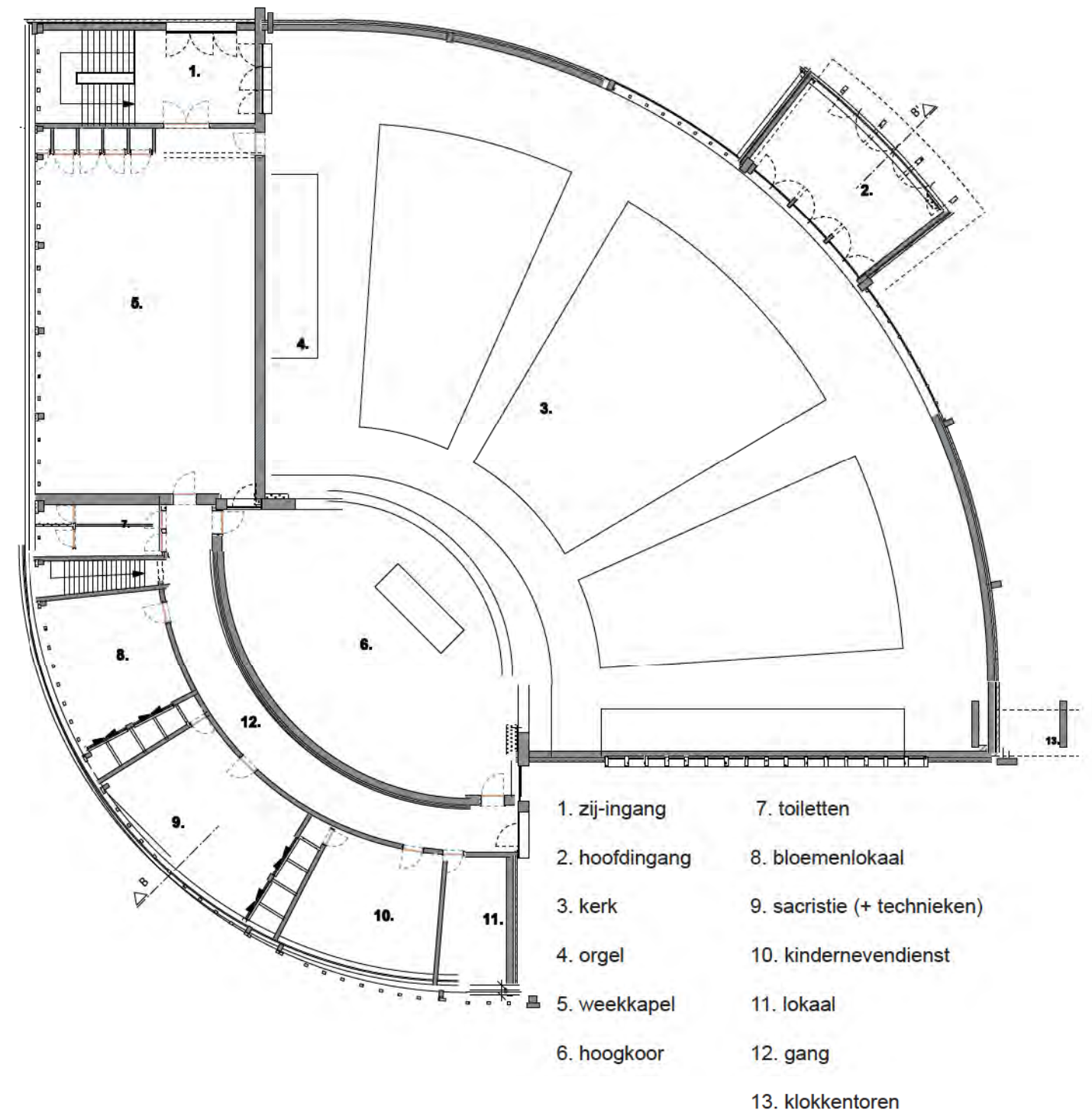
GELIJKVLOERS BESTAAND
