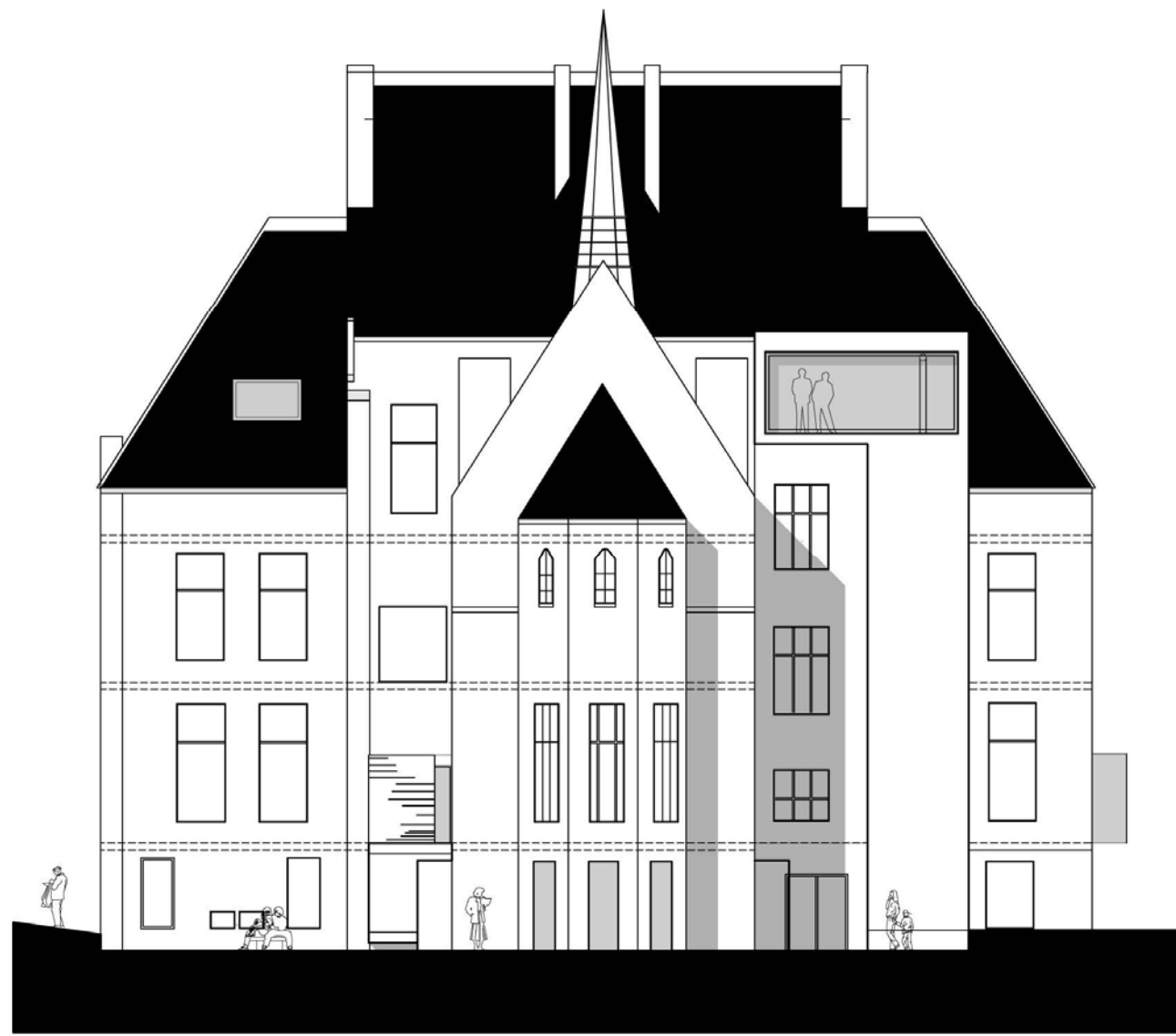
NOORDGEVEL
