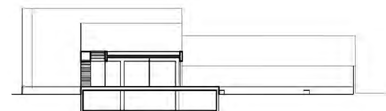
Snede CC
