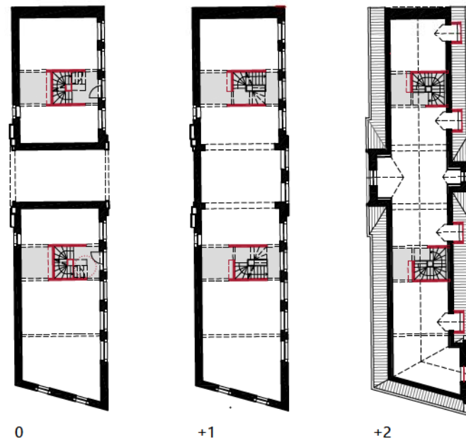
Varianten Poortgebouw: links generische plattegrond + rechts invulling met 7 gastenverblijven voor 8 personen (onderaan op 0 een verblijf met 2 slaapkamers)
