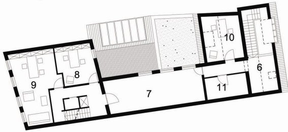
Eerste verdiep
