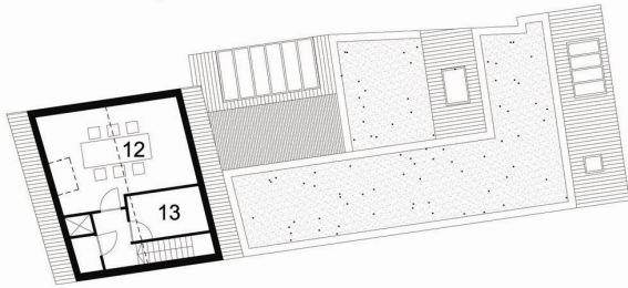
Tweede verdiep
