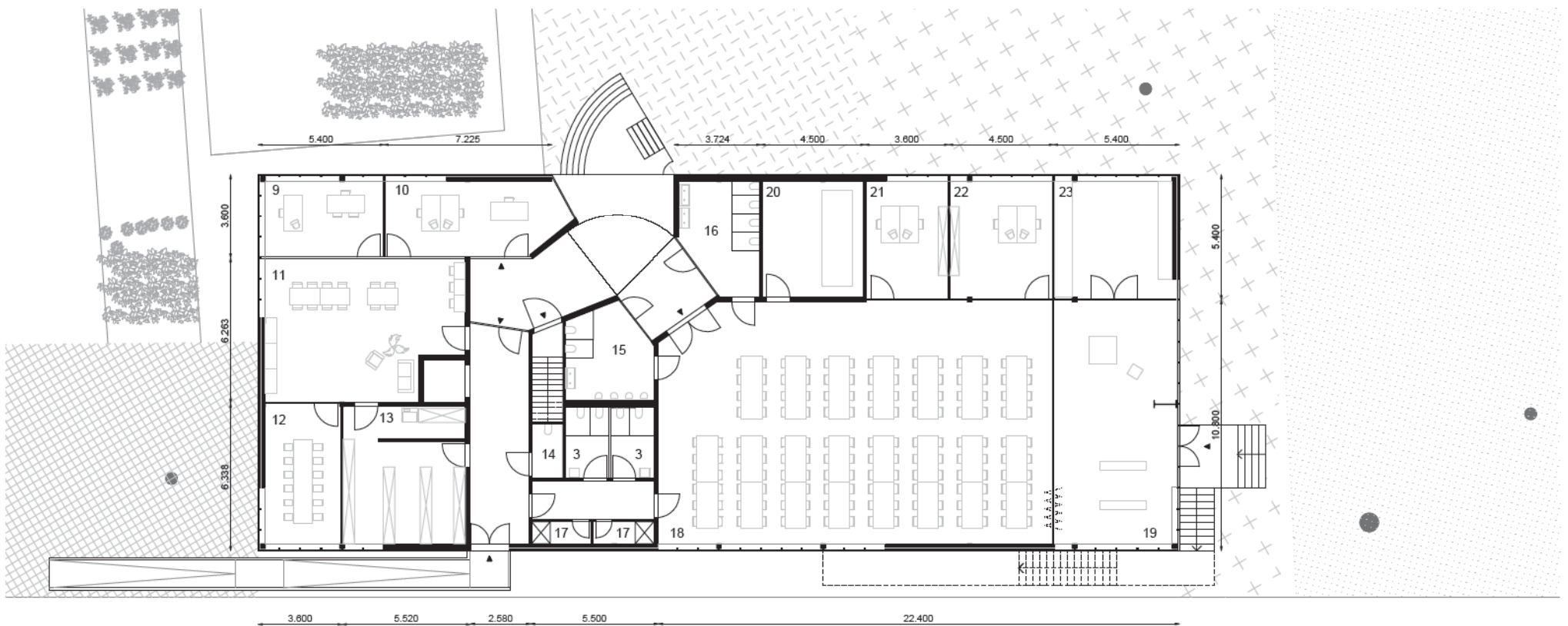
PLAN GELIJKVLOERS
