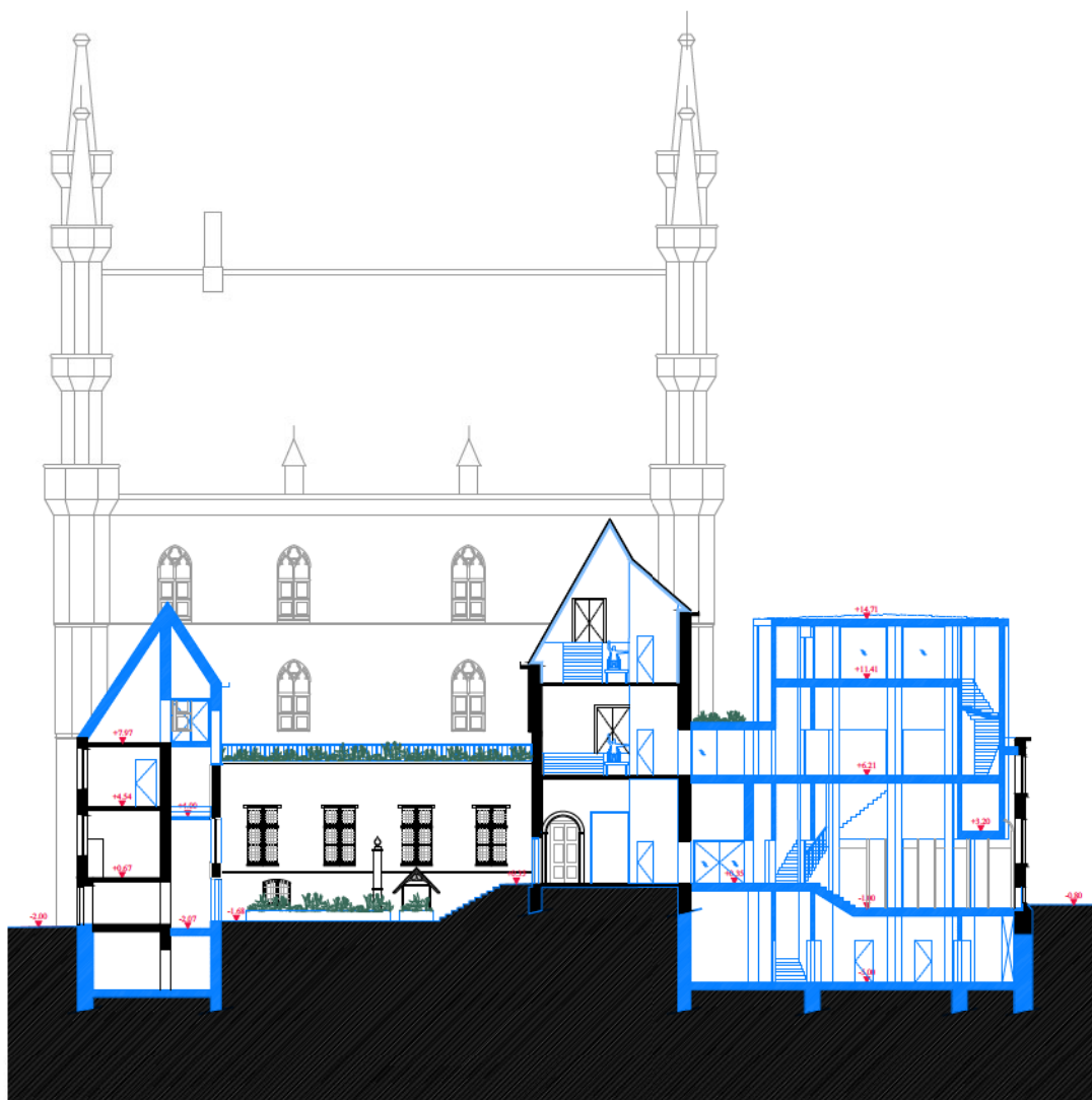
Snede Achterhuis - Antichambre: drenpelloze verbindingen
